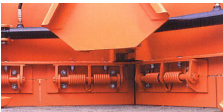
Federklappe mit Kunststoffschürfleiste
